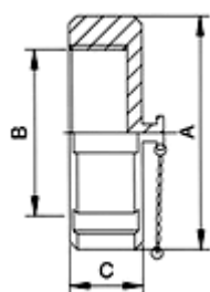
SMS-13RBN Blank Nut
