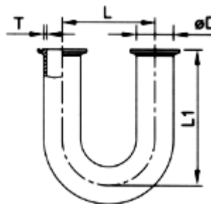
BPE 180° U-Joint Clamp End (DT-24)
