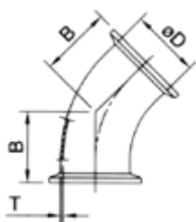
BPE 45° Elbow Clamp End (DT-17)
