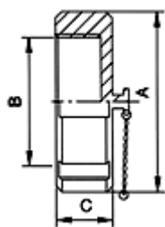
DANSK-13BR Blank Nut
