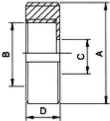
IDF-13R Round Nut
