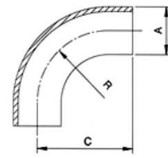
2S 90° Long Elbow
