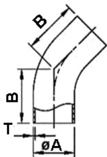
BPE 45° Elbow Weld End (DT-8)
