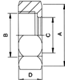
RJT-13H Hex. Nut
