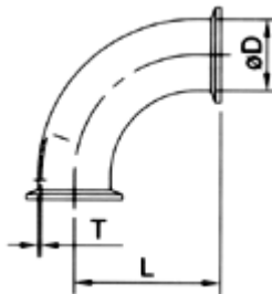
BPE 90° Elbow Clamp End (DT-16)
