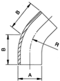
DIN 45° Long Elbow
