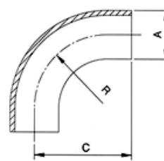
DIN 90° Long Elbow
