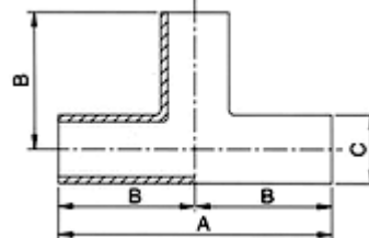
7W Long Equal Tee
