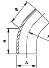
BS 45° Long Elbow
