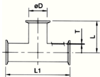
BPE Equal Tee Clamp End (DT-18)
