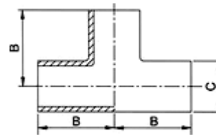
DIN Equal Tee
