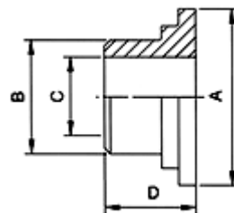
DANSK-14F Welding Liner
