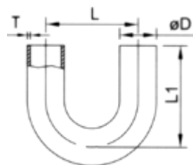
BPE 180° U-Joint Weld End (DT-23)
