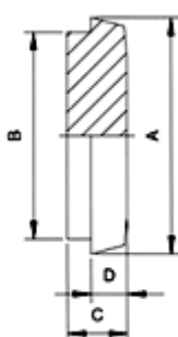
DIN-16(DIN-11851) Blank
