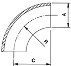
DIN 90° Short Elbow
